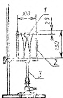
1 — тигель, 2 — асбестовые трубки толщиной 5 мм; 3 — горелка Теклю
