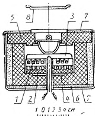
Электронагревательная печь
