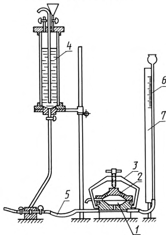
1 — резервуар для воды; 2 — кольцевой зажим; 3 — струбина; 4 — стеклянный цилиндр; 5 — резиновые трубки; 6 — водяной манометр; 7 — штатив
