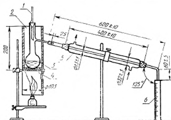
1—термометр; 2, 4—металлические кожухи; 3—колба; 5—холодильник; 6—цилиндр
