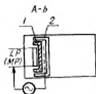
1 — ОСНОВНАЯ ИЗОЛЯЦИЯ; 2 — ДОПОЛНИТЕЛЬНАЯ ИЗОЛЯЦИЯ
