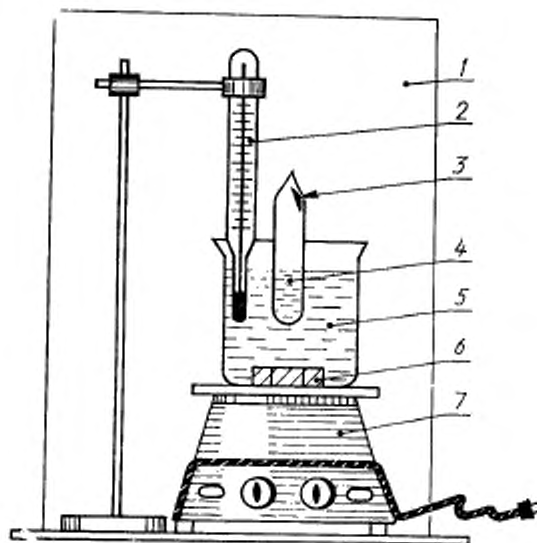
1—защитный экран; 2—термометр; 3—зажимная ампула; 4—исследуемый раствор; 5—теплопроводящая жидкость; 6—мешалка; 7—нагревательный прибор
