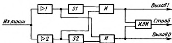
Схема распознавания импульсов
