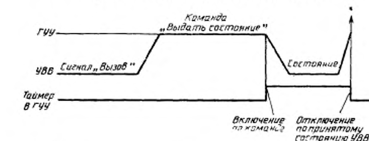
Временная диаграмма обработки сигнала «Вызов»
