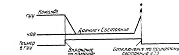
Временная диаграмма для команд чтения
