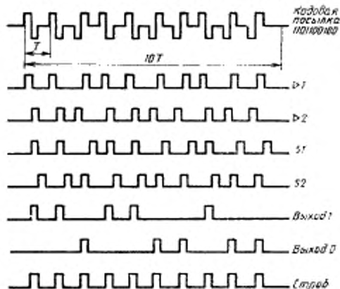
Временная диаграмма разделения импульсов
