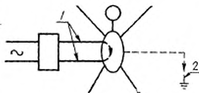
Рис. 2. Ток утечки на пациента 1 — наглядываемая часть или цепь пациента; 2 — ток утечки
