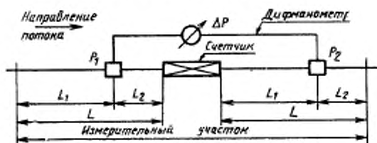
Схема измерительного участка
