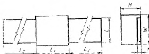
Черт. 7
