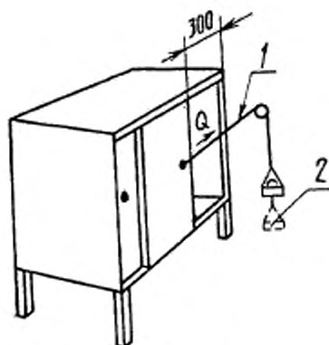
1—трос; 2—груз
