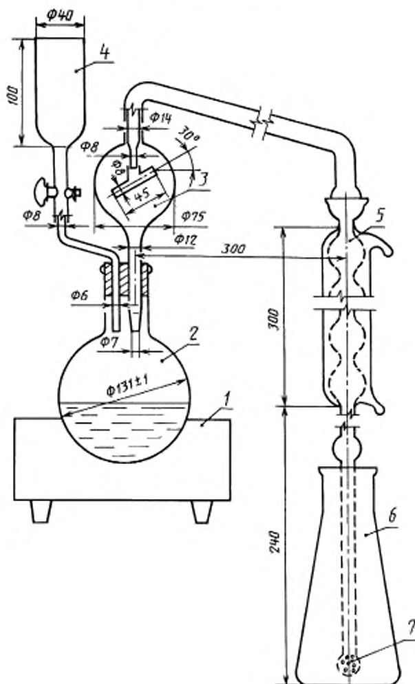
1 — колба-нагреватель; 2 — реакционная колба вместимостью 0,5—1,0 дм 3 ; 3 — каплеуловитель; 4 — капельная воронка с краном; 5 — холодильник; 6 — приемник; 7 — барбатор
