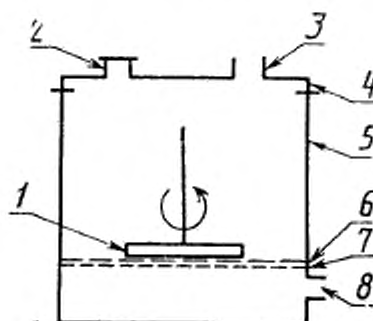
1—магнитная мешалка; 2—предохранительный клапан; 3—патрубок подачи давления; 4—крышка; 5—корпус; 6—испытуемый образец мембраны; 7—дренаж; 8—отверстие для выпуска фильтрата
