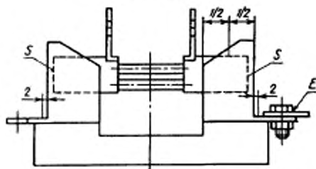
Черт. 7 (П). Испытательный нож по п. 8.5.5.1.2
