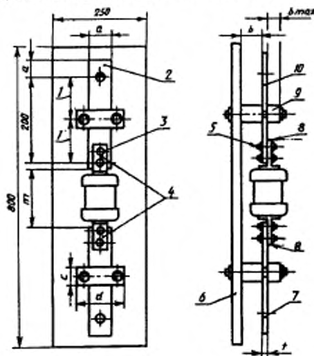
Черт. 5 (II). Устройство для испытаний на потери мощности
