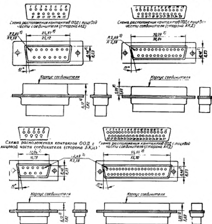
Рисунок 4.1 — Соединитель ООД
