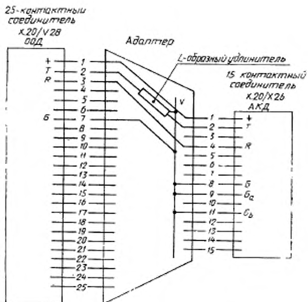
+) См. своску 1) к таблице 1 Рисунок С.4 — Схема монтажа адаптера
