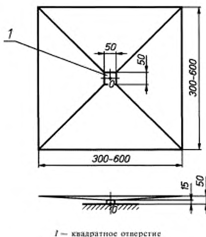
Рисунок 3.2 — Испытательное устройство для дорожного просвета
