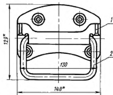
Ручка 2 ОКП 72898 84302
