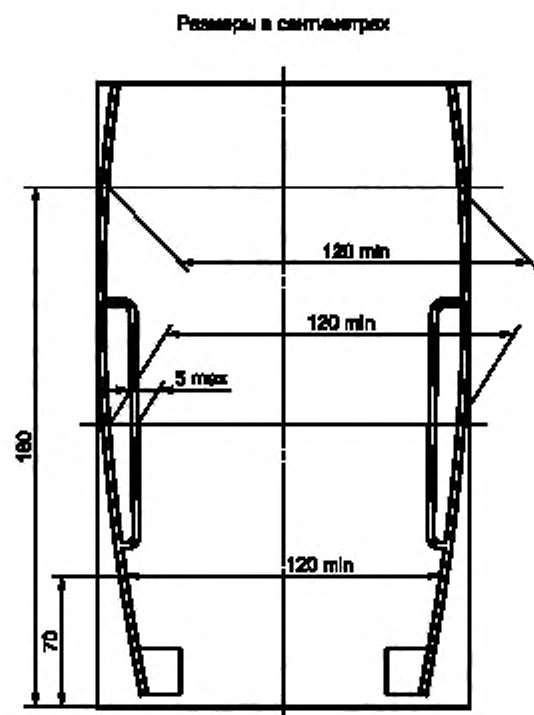
Рисунок Г.12 — Пром служебной двери. Сдвоенная дверь (см. 5.6.3.1)
