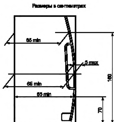
Рисунок Г.13 — Пром служебной двери. Одинарная дверь (см. 5.6.3.1)
