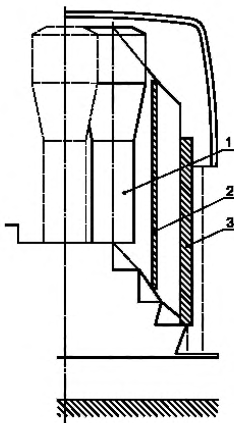
1 — цилиндрический шаблон; 2 — вертикальный шаблон, 3 — двойной шаблон
