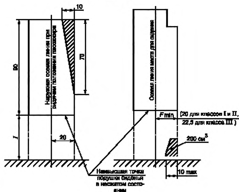
Рисунок Г.10 — Допустимый выступ элемента конструкции (см. 5.7.8.6.2.2)
