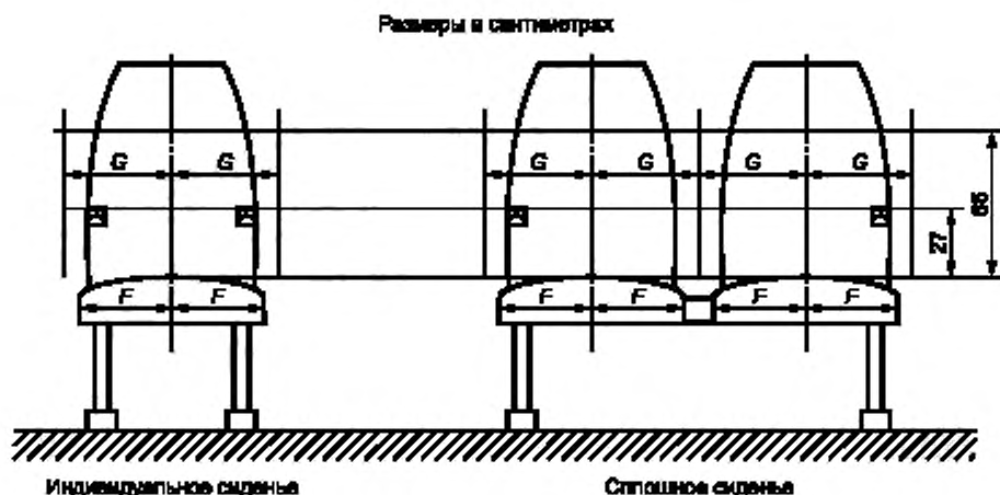
Рисунок Г.5 — Ширина пассажирских сидений (см. 5.7.8.1)
