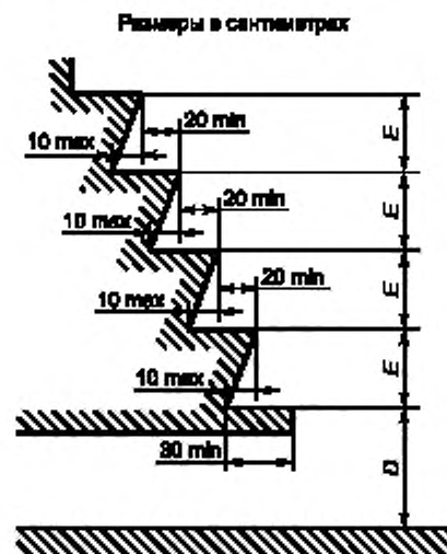
Рисунок Г.4 — Ступеньки для пассажиров (см. 5.7.7)
