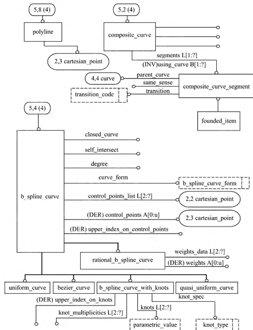
Рисунок С.5 — alc_geometrically_bounded_2d_wireframe — EXPRESS-G диаграмма 5 из 5
