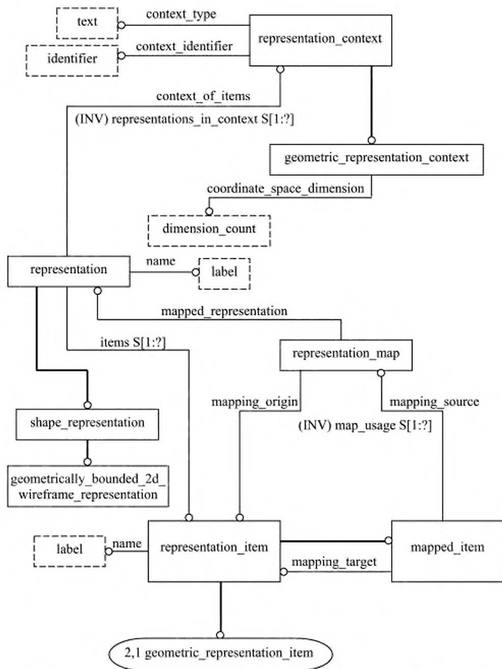
Рисунок С.1 — alic_geometrically_bounded_2d_wireframe — EXPRESS-G диаграмма 1 из 5
