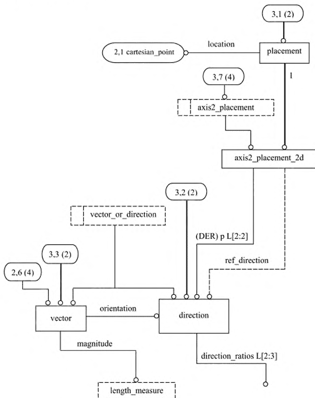
Рисунок С.3 — aic_geometrically_bounded_2d_wireframe — EXPRESS-G диаграмма 3 из 5
