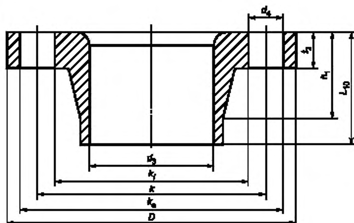
Рисунок 6 — Размеры фланцевой втулки
