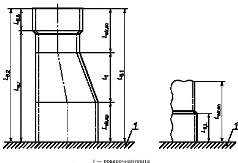
Рисунок 5 — Определение эффективной длины перехода
