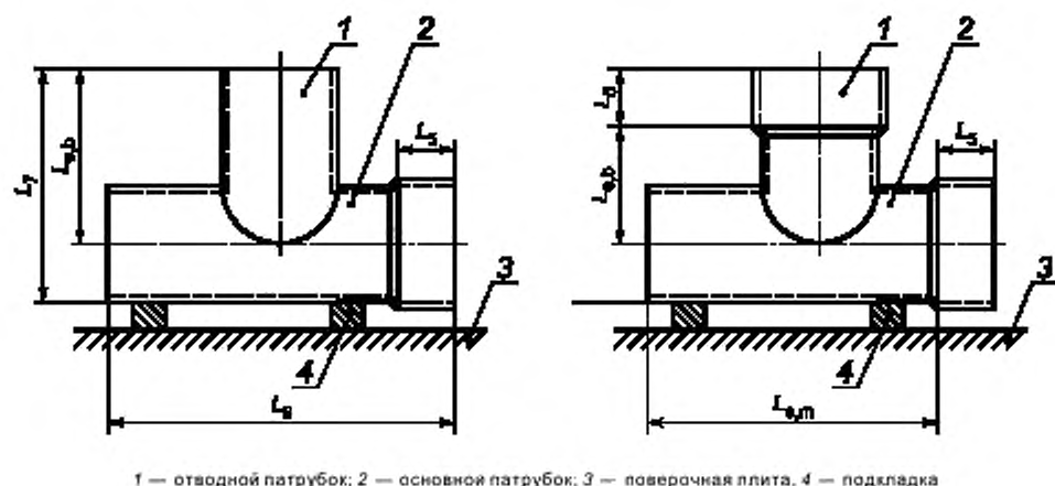
Рисунок 3 — Определение длин тройника
