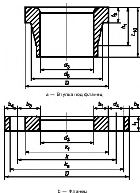
Рисунок 7 — Размеры втулки под фланец и фланца
