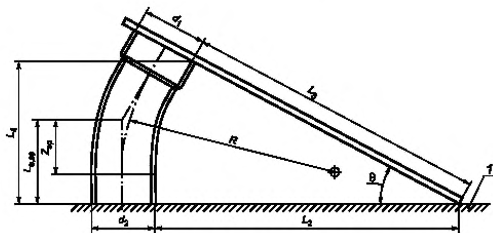
б — Отвод установлен на трубный конец
