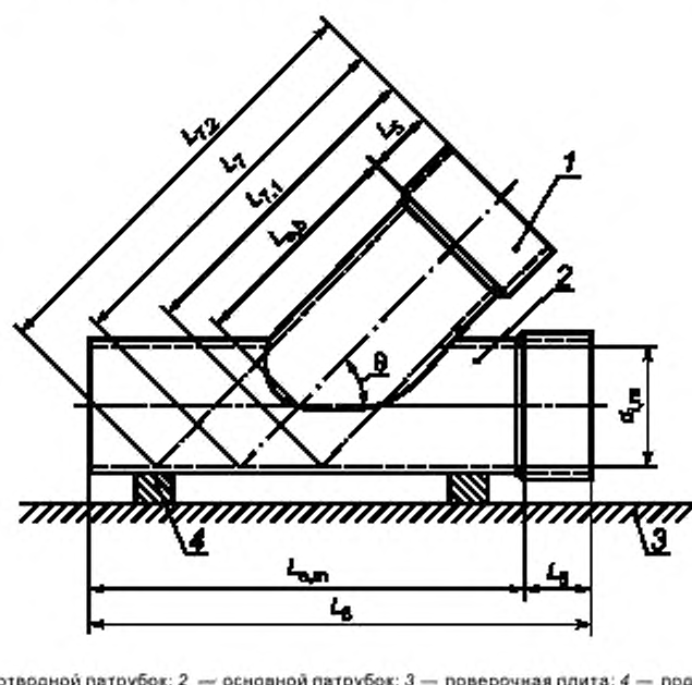
Рисунок 4 — Определение эффективной длины отводного патрубка тройника, расположенного под углом, отличным от 90°
