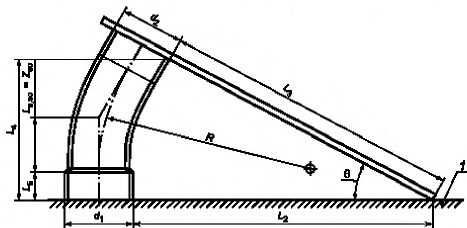
а — Отвод установлен на конец с раструбом
